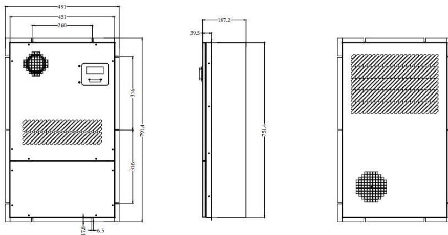
Рисунок 4 – Габаритные размеры SNR-ACC-1000-DCH и SNR-ACC-1500-DCH
