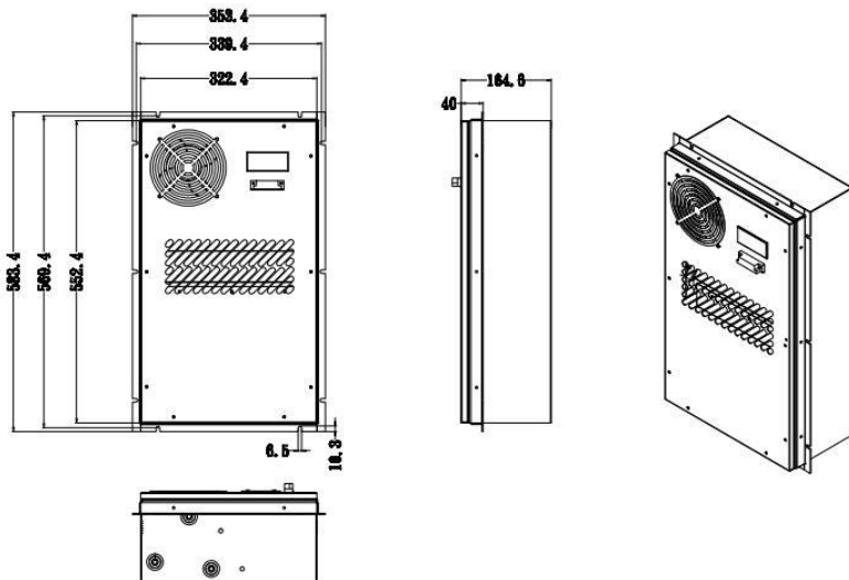
Рисунок 3 – Габаритные размеры SNR-ACC-500-DCH.V2
