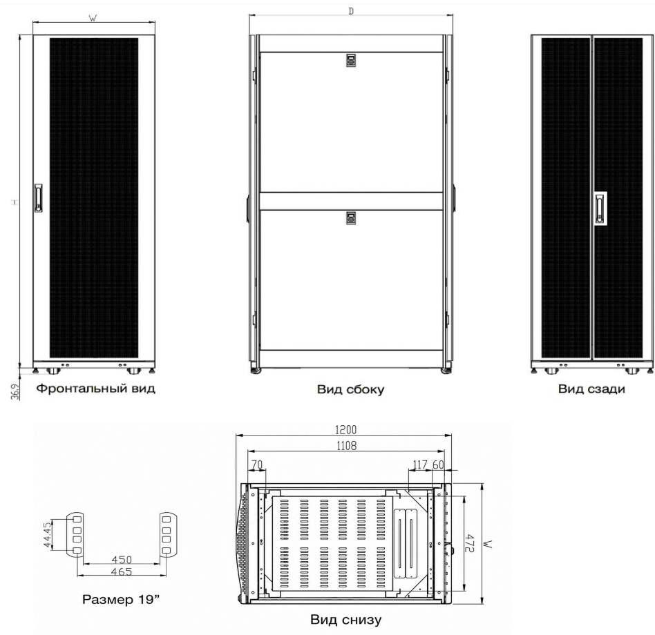
Рисунок 3 – Габаритные размеры шкафа
