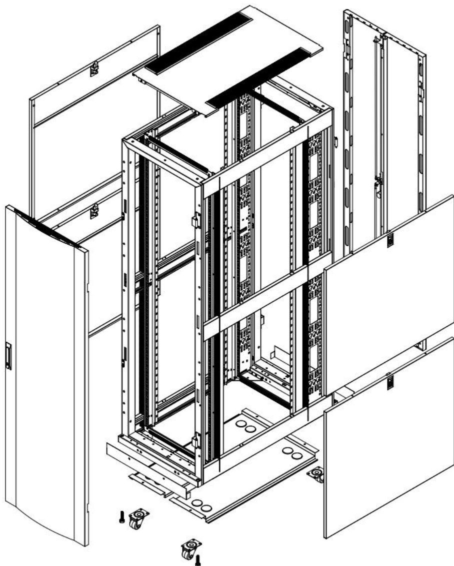
Рисунок 1 – Комплектация шкафа
