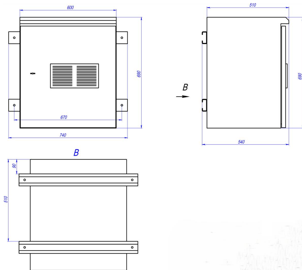
Рисунок 2 – Габаритные размеры
