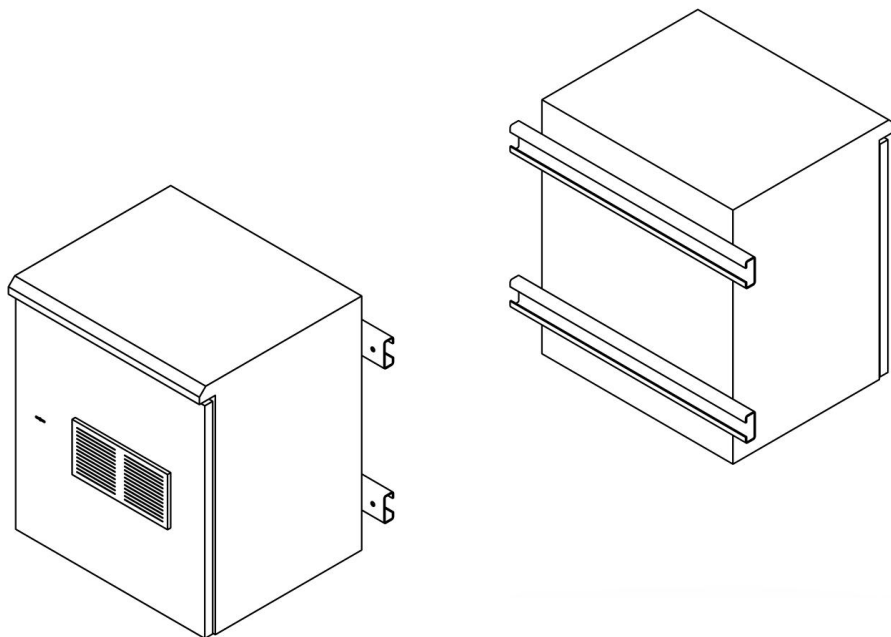
Рисунок 1 – Общий вид
