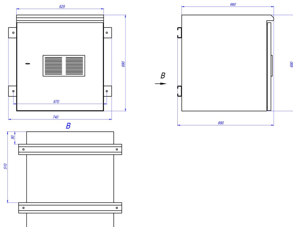
Рисунок 2 – Габаритные размеры
