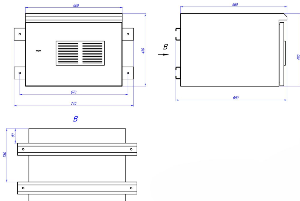
Рисунок 2 – Габаритные размеры
