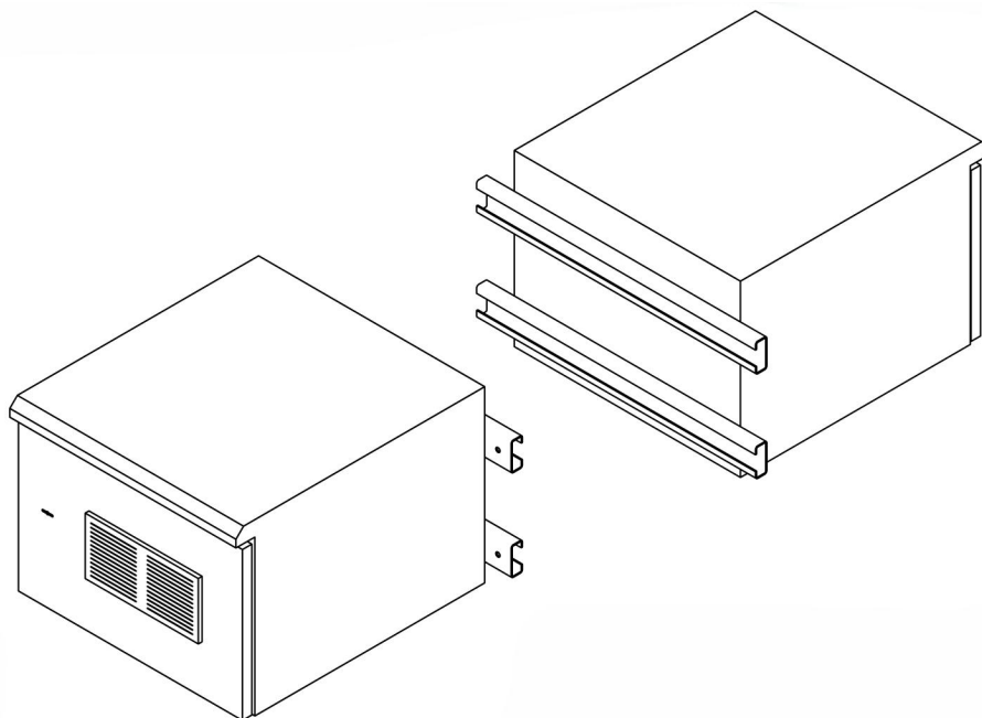
Рисунок 1 – Общий вид
