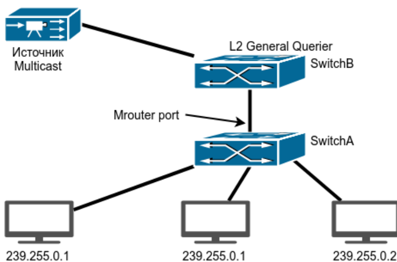
Рис. 31: IGMP Querier
