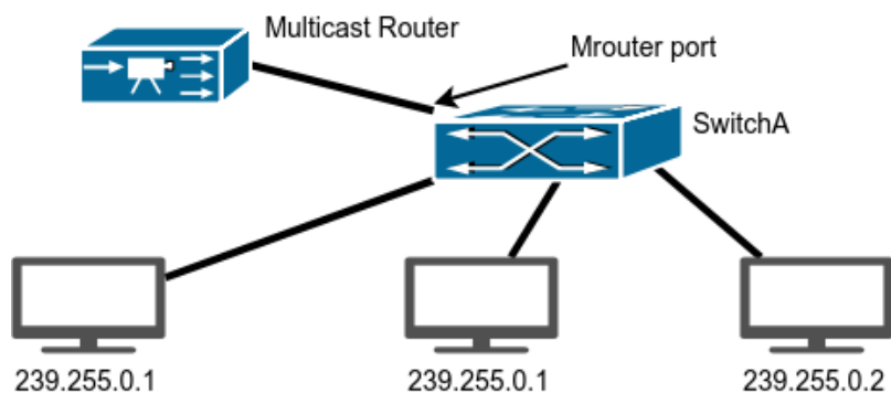
Рис. 30: IGMP Snooping
