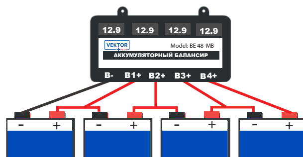
рис. 1 Банк батарей на 48 В из 4-х АБ
