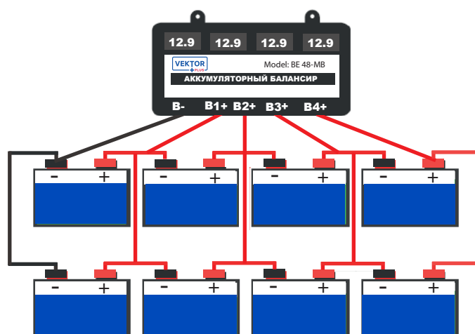
рис. 2 Банк батарей на 48 В из 8-ми АБ
